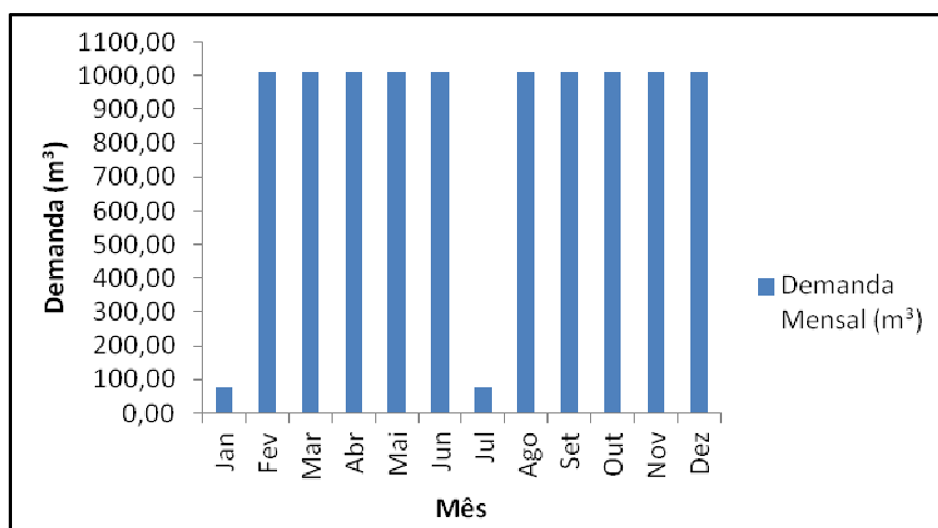
Figura 8 - Consumo de água não potável em meses letivos e férias
